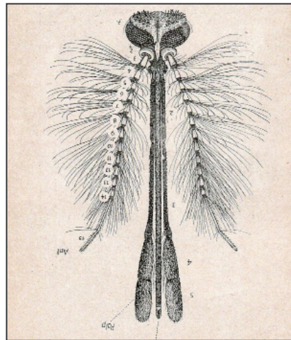
Abb. 1 Mückenkopf, männlich
